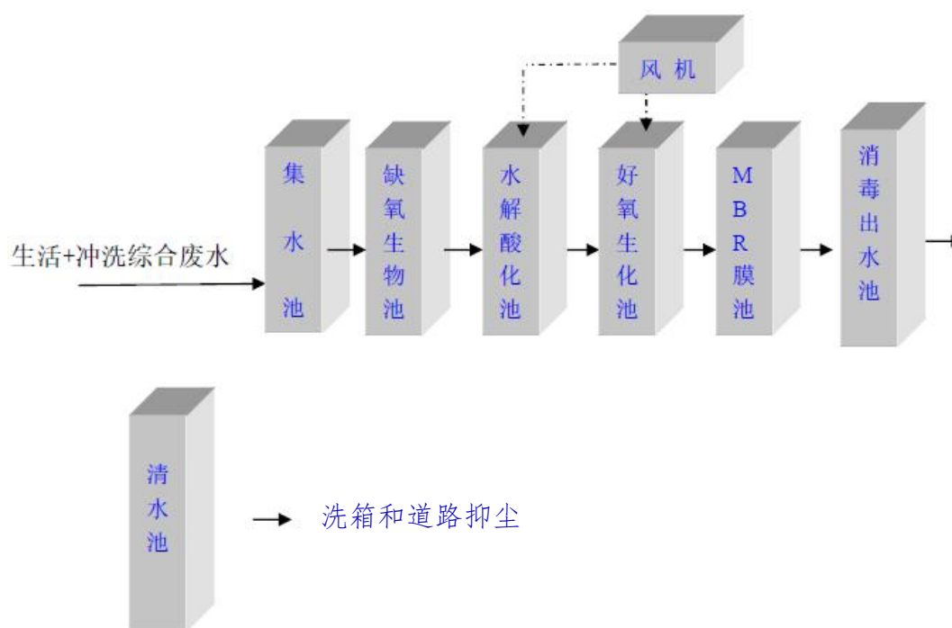
图 2.5-1 污水处理工艺流程图
