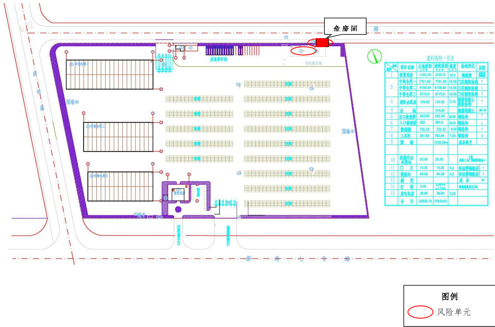
附图 1 企业平面布置及风险单元分布图
